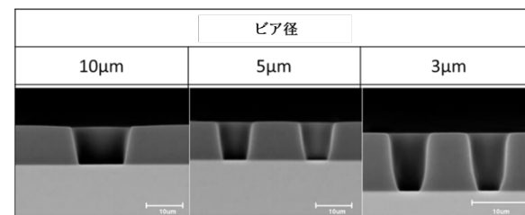
ZC100の解像度 (厚さ: 10μm、硬化温度: 180℃)
